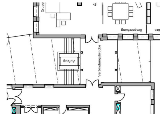
GRUNDRISS OBERGESCHOSSE
