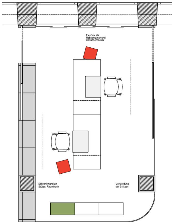
DOPPELBÜRO
