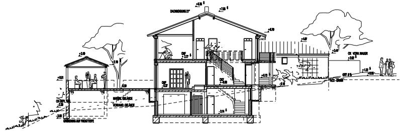
SCHNITT A-A
